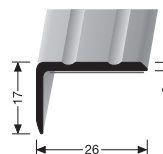
237 SK TREPPENWINKEL ANGLE EDGE
