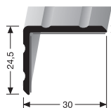
234 SK TREPPENWINKEL ANGLE EDGE
