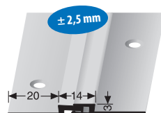
317 SK BEWEGUNGSFUGENPROFIL MOVEMENT JOINT PROFILE
