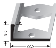
303 G DOPPEL-K PROFIL DOUBLE K PROFILE
