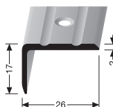
237 TREPPENWINKEL ANGLE EDGE
