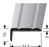
236 SK TREPPENWINKEL ANGLE EDGE
