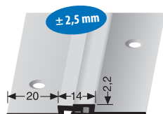
316 SK BEWEGUNGSFUGENPROFIL MOVEMENT JOINT PROFILE
