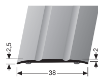
438 SK ÜBERGANGSPROFIL TRANSITION PROFILE
