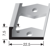
307 G DOPPEL-K PROFIL DOUBLE K PROFILE
