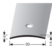
459 ÜBERGANGSPROFIL TRANSITION PROFILE
