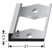
301 G DOPPEL-K PROFIL DOUBLE K PROFILE
