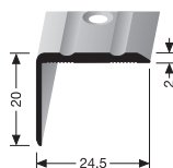
235 TREPPENWINKEL ANGLE EDGE
