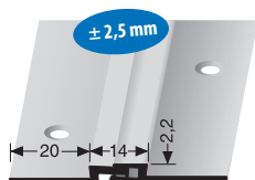
316 BEWEGUNGSFUGENPROFIL MOVEMENT JOINT PROFILE
