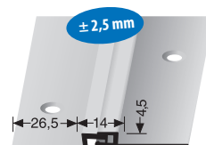
318 SK BEWEGUNGSFUGENPROFIL MOVEMENT JOINT PROFILE
