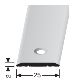
442 ÜBERGANGSPROFIL TRANSITION PROFILE
