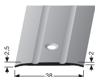
438 ÜBERGANGSPROFIL TRANSITION PROFILE
