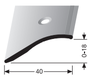
248 ABSCHLUSSPROFIL EDGE TRIM
