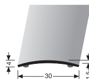
459 SK ÜBERGANGSPROFIL TRANSITION PROFILE
