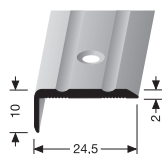
236 TREPPENWINKEL ANGLE EDGE
