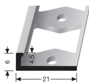
302 G DOPPEL-K PROFIL DOUBLE K PROFILE
