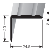
235 SK TREPPENWINKEL ANGLE EDGE
