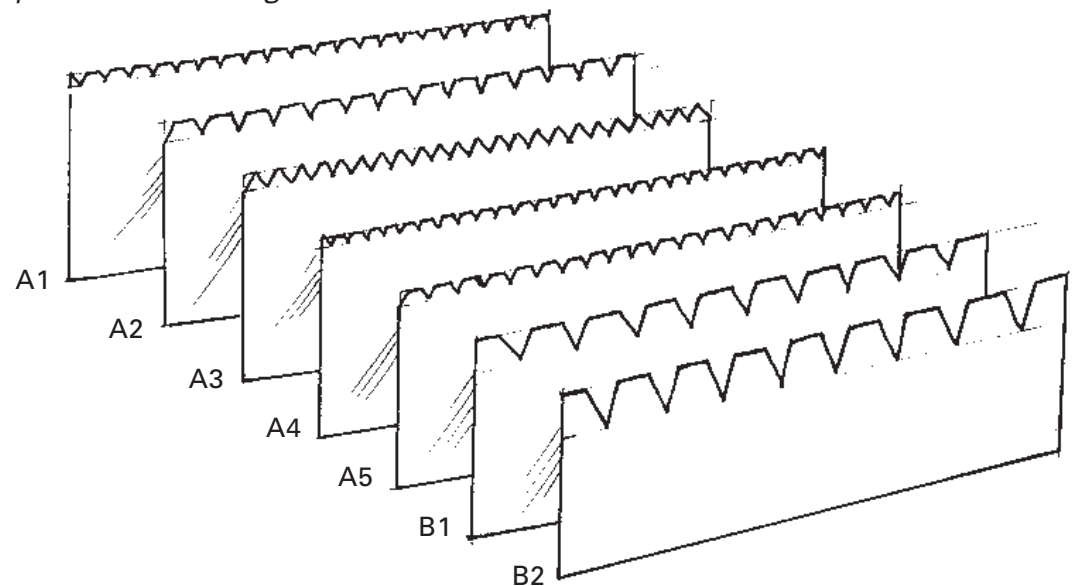
Klebstoff-Spachtelzahnungen
