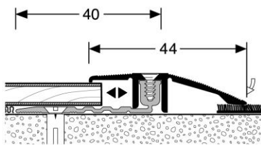
Anpassungsprofil 486
