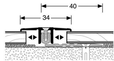
Übergangprofil 488
