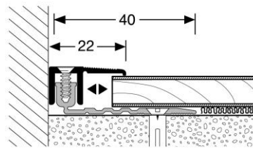
Abschlussprofil 487
