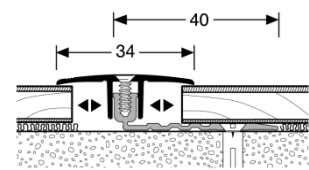
Übergangprofil 289
