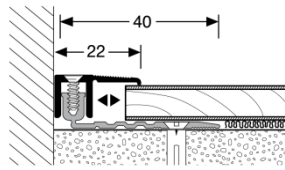
Abschlussprofil 287
