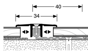
Übergangprofil 288
