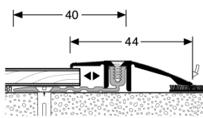
Anpassungsprofil 286
