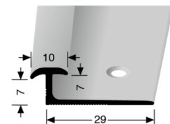
Profil 297 V
