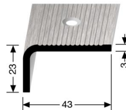
Profil 545 V
