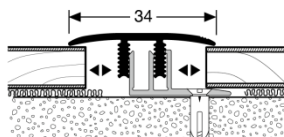
Profil 568
