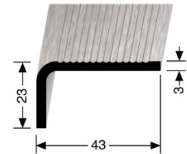
Profil 545 U
