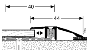
Anpassungsprofil 286
