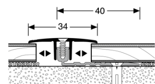
Übergangprofil 289
