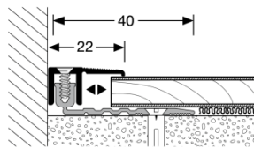
Abschlussprofil 287
