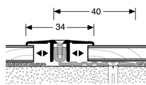
Übergangprofil 288
